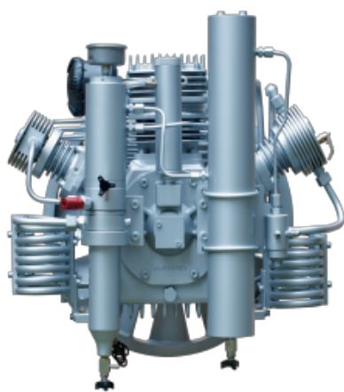
W-max. 350Bar
